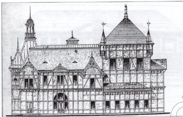
A faszínház oldalnézete
